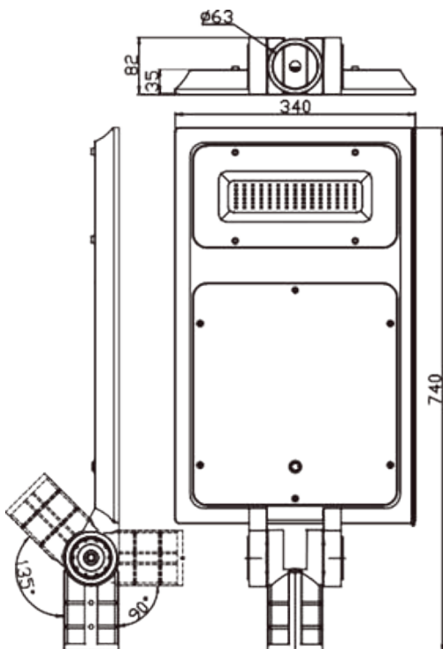
SLSYS40W
