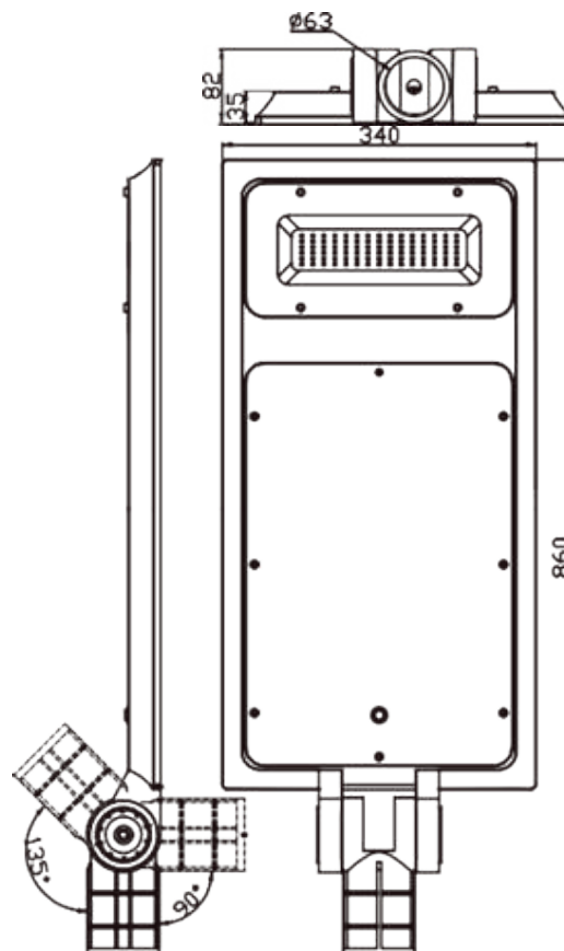
SLSYS60W
