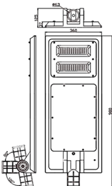
SLSYS100W
